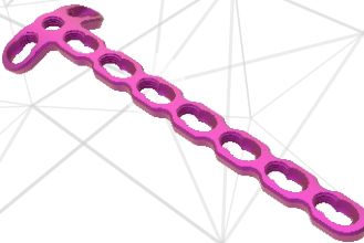
2.0 mm Mini T Locking Plate
